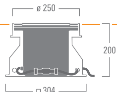
ETC339-FS
