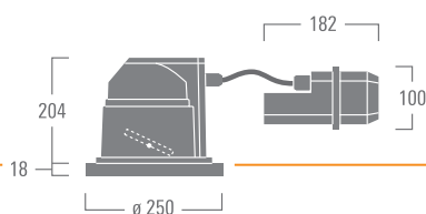
DOC240-GB
