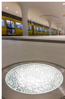
08 An den Bahnsteigenden sind ETC140 Bodeneinbauleuchten mit 24 LED in 3000 K installiert und mit rutschhemmender Keramikbeschichtung „ASC“ nach DIN 51130 versehen.
